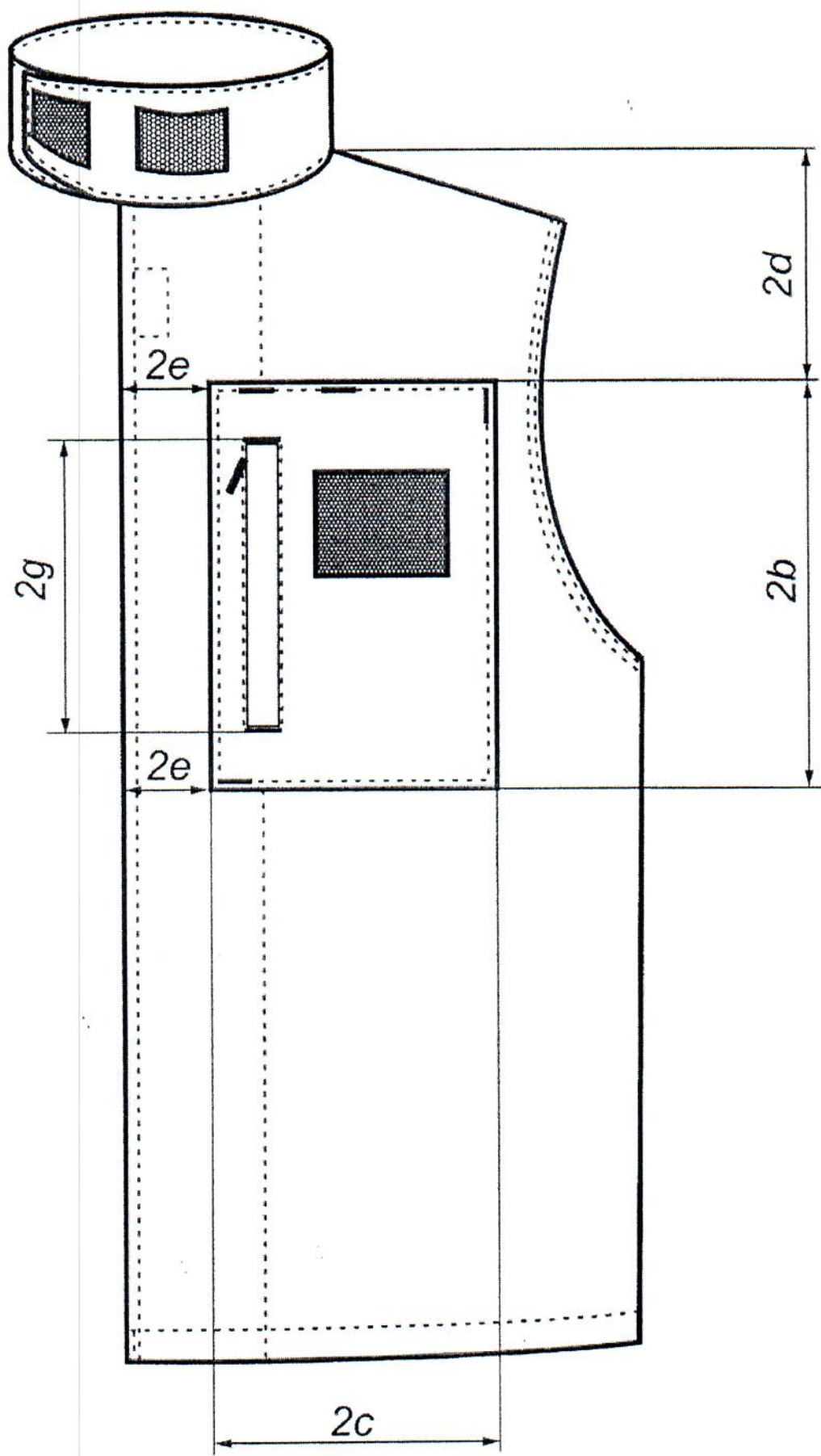
Rysunek 3 – Przód bluzy rozmieszczenie kieszeni
